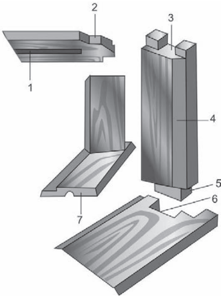
Рис. 4.15. Устройство коробки: 1 — вершиник; 2, 5 — шип; 3, 6 — проушина; 4 — стояк, 7 — слезник
