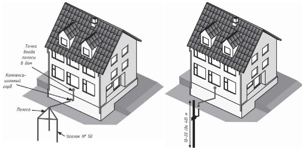
Рис. 8.16. Заземлитель и соединение его с главной заземляющей шиной в здании. Сборный штырь можно углубить в грунт на 20–40 м
