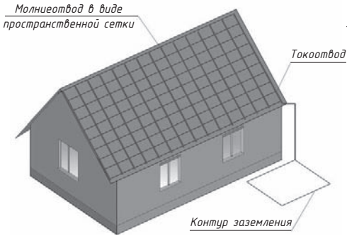
Рис. 8.14. Молниеотвод на основе «пространственной сетки»
