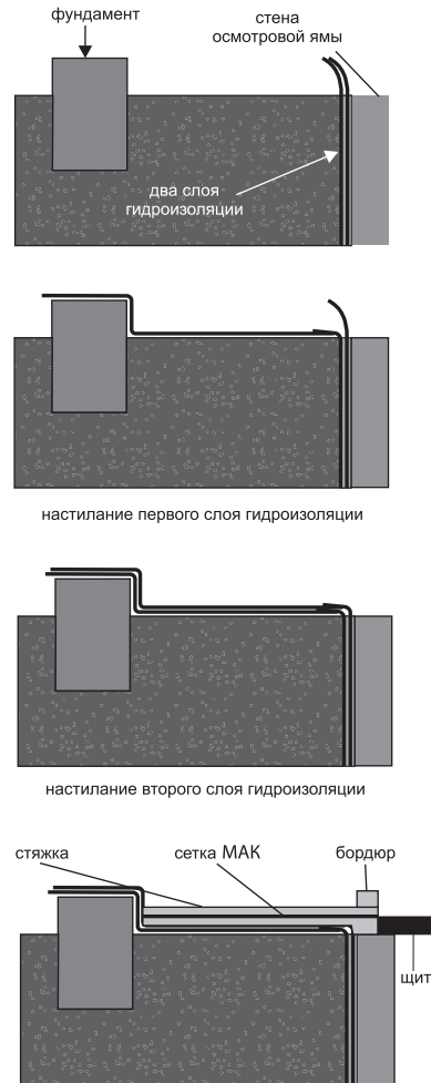
Рис. 13.6. Устройство стяжки
