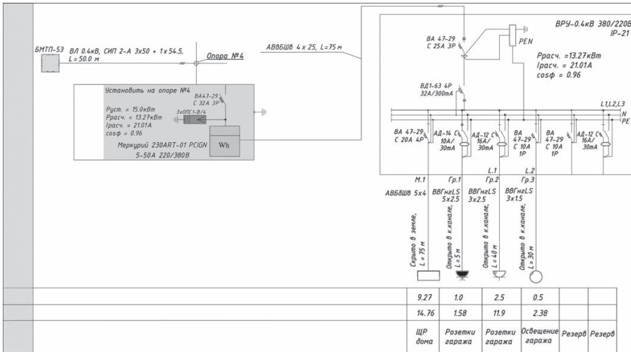
Рис. 8.3. Однолинейная схема
