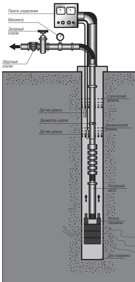
Рис. 9.13. Схема погружного насоса
