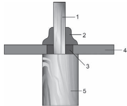
Рис. 4.8. Установка перегородки на балку: 1 — перегородка; 2 — плинтус; 3 — брусок; 4 — пол; 5 — балка
