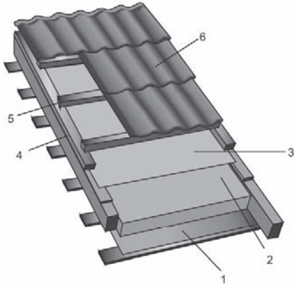
Рис. 5.27. Схема крыши деревянного дома с отапливаемым чердаком или мансардным этажом: 1 — пароизоляция; 2 — утеплитель (минеральная вата); 3 — ветровлагозащитная мембрана; 4 — контробрешетка; 5 — поперечная обрешетка; 6 — черепица
