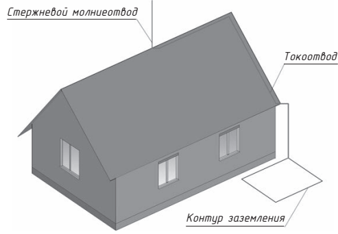
Рис. 8.13. Стержневой молниеотвод
